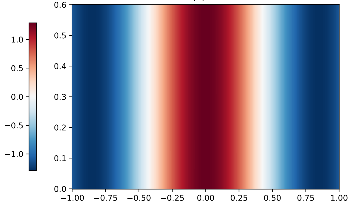
Re(u) PINN
